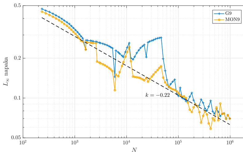
Slika 24: Konvergenca metode pri reševanju Hertzevega kontaktnega problema (4.24).
