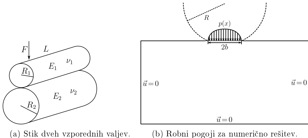
Slika 22: Obravnavan Hertzjev kontaktni problem.
