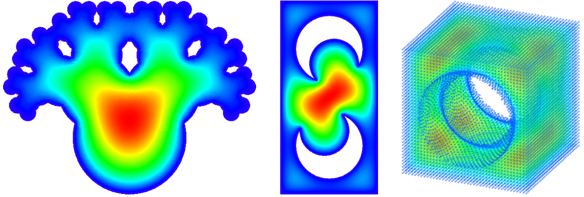
Slika 17: Reševanje Poissonove enačbe \Delta u = 1 s homogenimi robnimi pogoji na zanimivejših domenah.
