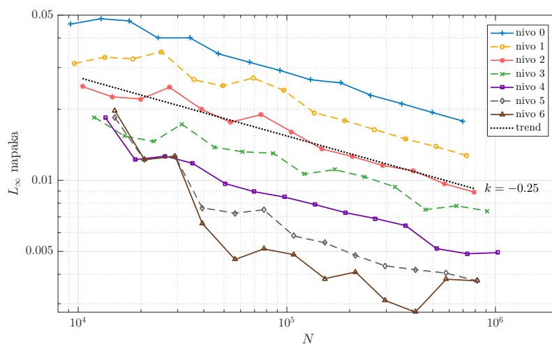
Slika 27: Napaka metode pri različnih nivojih sekundarnega zgoščevanja.
