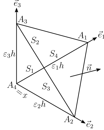
Slika 3: Tetraeder, uporabljen v dokazu Cauchyjevega izreka o napetosti.
