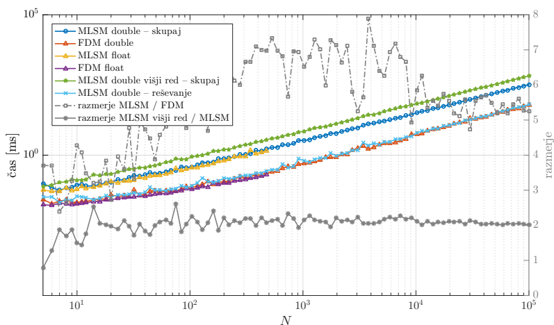
Slika 12: Primerjava časa izvajanja MLSM in FDM metod.
