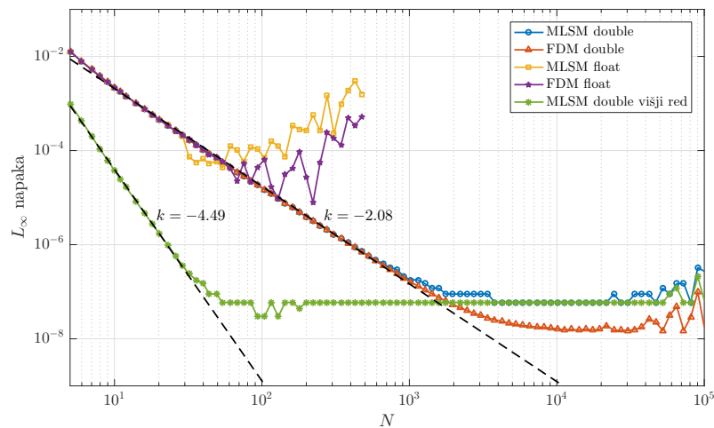
Slika 11: Napaka FDM in MLSM metode v primerjavi s pravilno rešitvijo.
