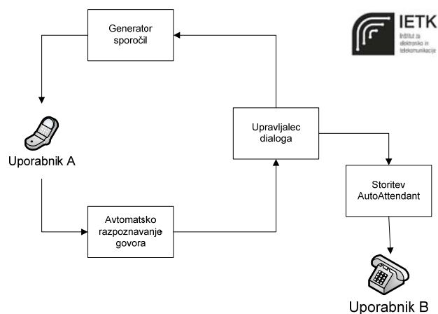
Slika 3. Projekt avtomatskega govorno vodenega telefonskega operaterja (AAT).
