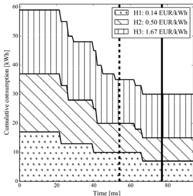
Slika 4. Primer uporabe mehanizma za določanje dinamičnih cen.
