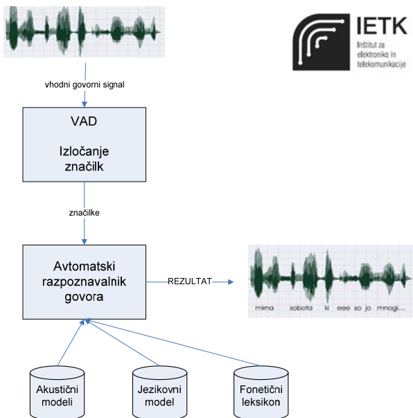
Slika 1. Blokovna shema avtomatskega razpoznavnika govora.
